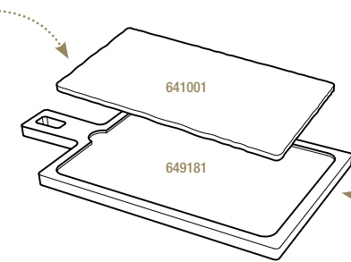
PLATEAU POUR ASSIETTE 30 x 20 cm LINER TRAY FOR PLATE 11 3/4 x 7 3/4"
